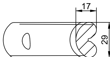
A-A (1:2)
