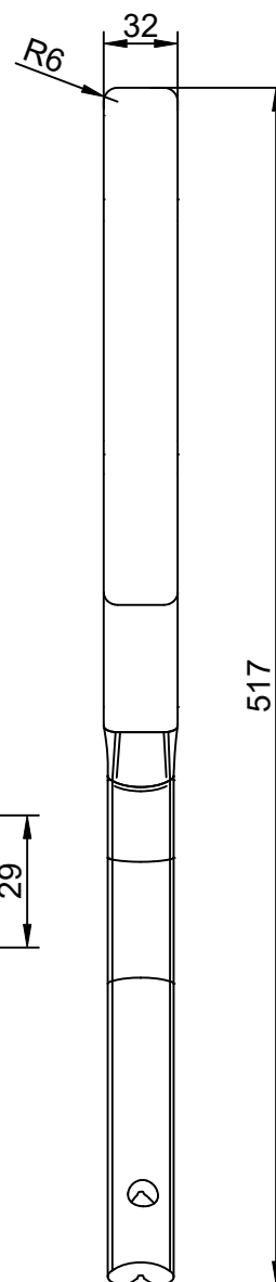
B-B (1:2)
