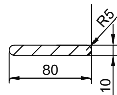
A-A (1:4)
