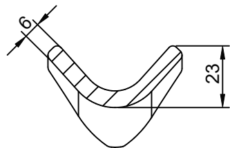
A-A (1:2)
