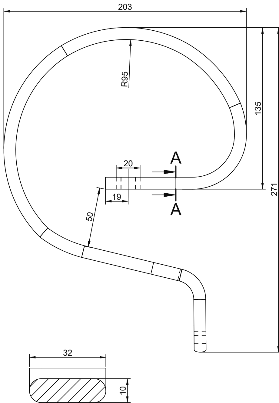
A-A (1:1)
