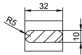
B-B (1:2)
