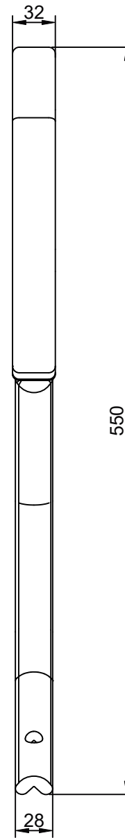
B-B (1:2)
