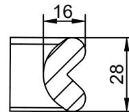
A-A (1:2)
